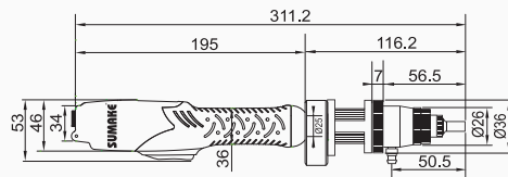
Lever Start Type EA-BN412LAS-D ~ EA-BN419LAS-D
