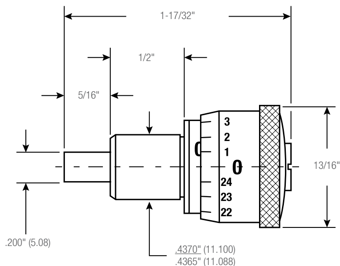
464P (0-1/4") dimensions
