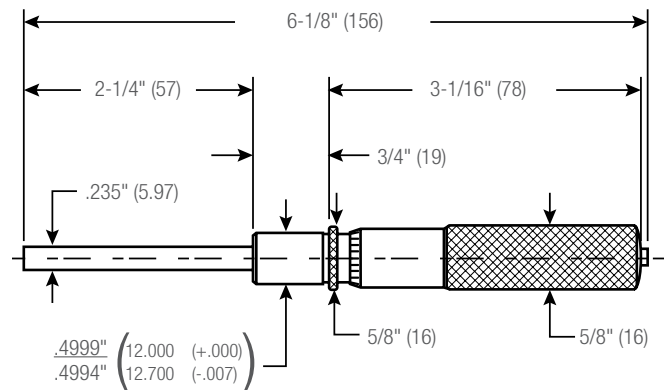
63P (0-2") and 63MP (0-50mm) dimensions
