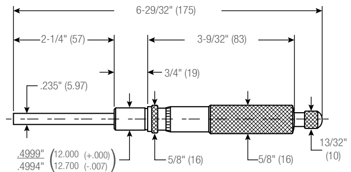
63RL (0-2") and 63MRL (0-50mm) dimensions
