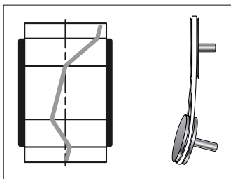
图8 显示同时存在三种不对中
