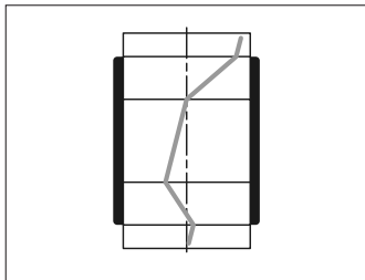
Рис 9 Шкивы с комбинацией трех несоосностей
