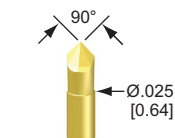
61 -S- Blade
