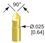
61 -S- Blade
