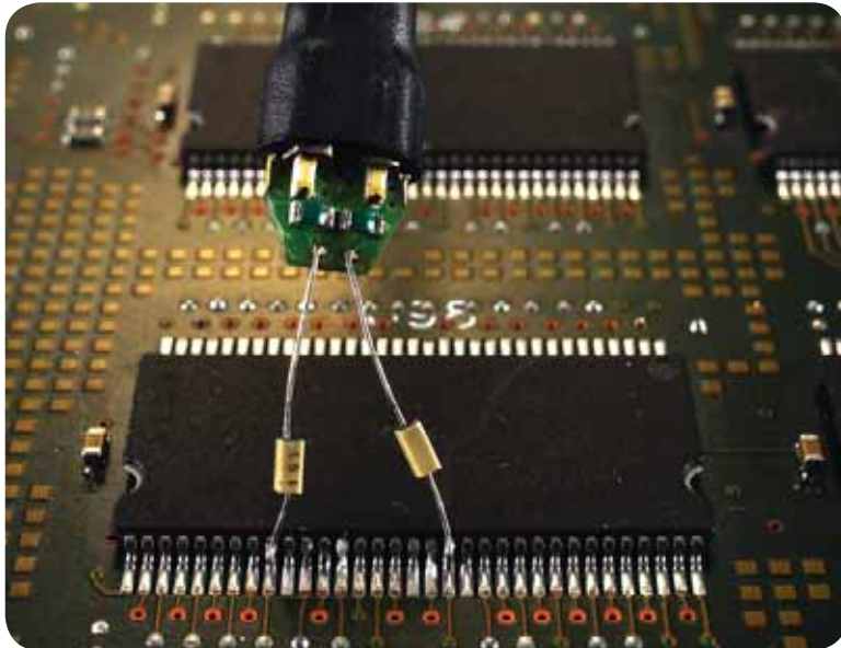
Figure 9: Long-wire ZIF tip
