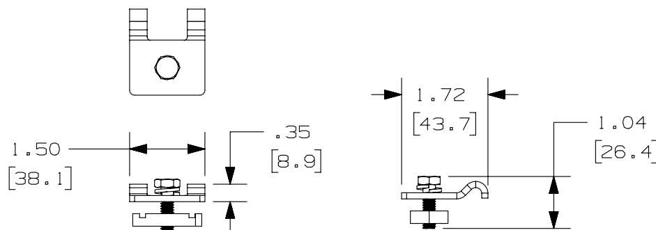
STRUT CLIP
