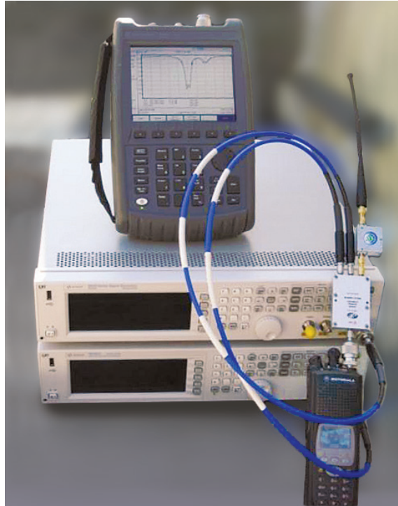
Figure 2. Actual test setup
