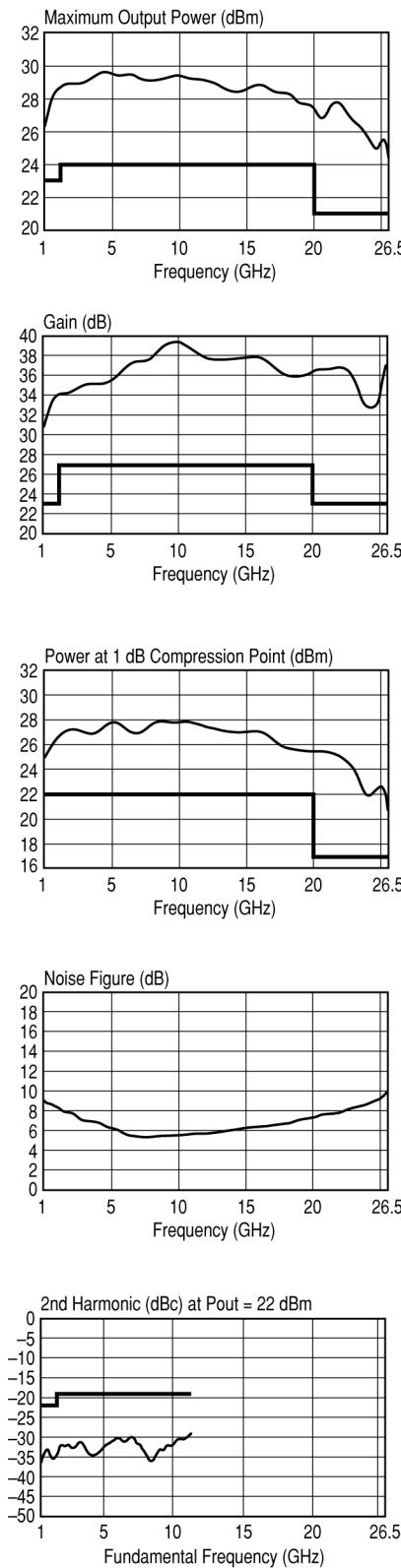
83018A Amplifier
