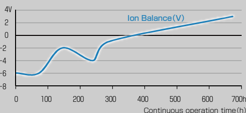
Ion balance(F-120R)
