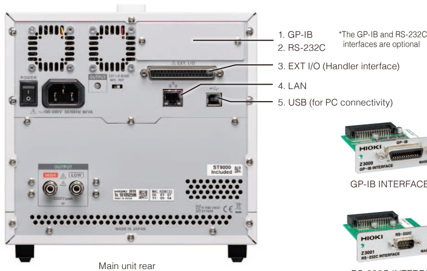
RS-232C INTERFACE Z3001
