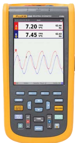
Fluke 125B
