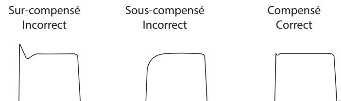
Figure 11: Compensation avec une forme d'onde HF
