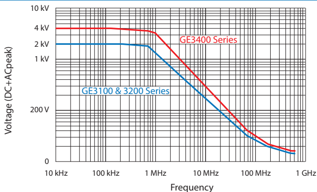
Abbildung 13: Spannungsderating-Kurve, GE3000 serie
