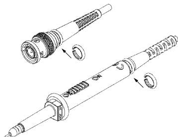
Figure 7: Fixer les bagues de couleur
