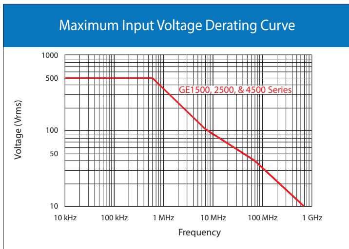
Abbildung 12: Spannungsderating-Kurve, GE1500, 2500, und 4500 serie
