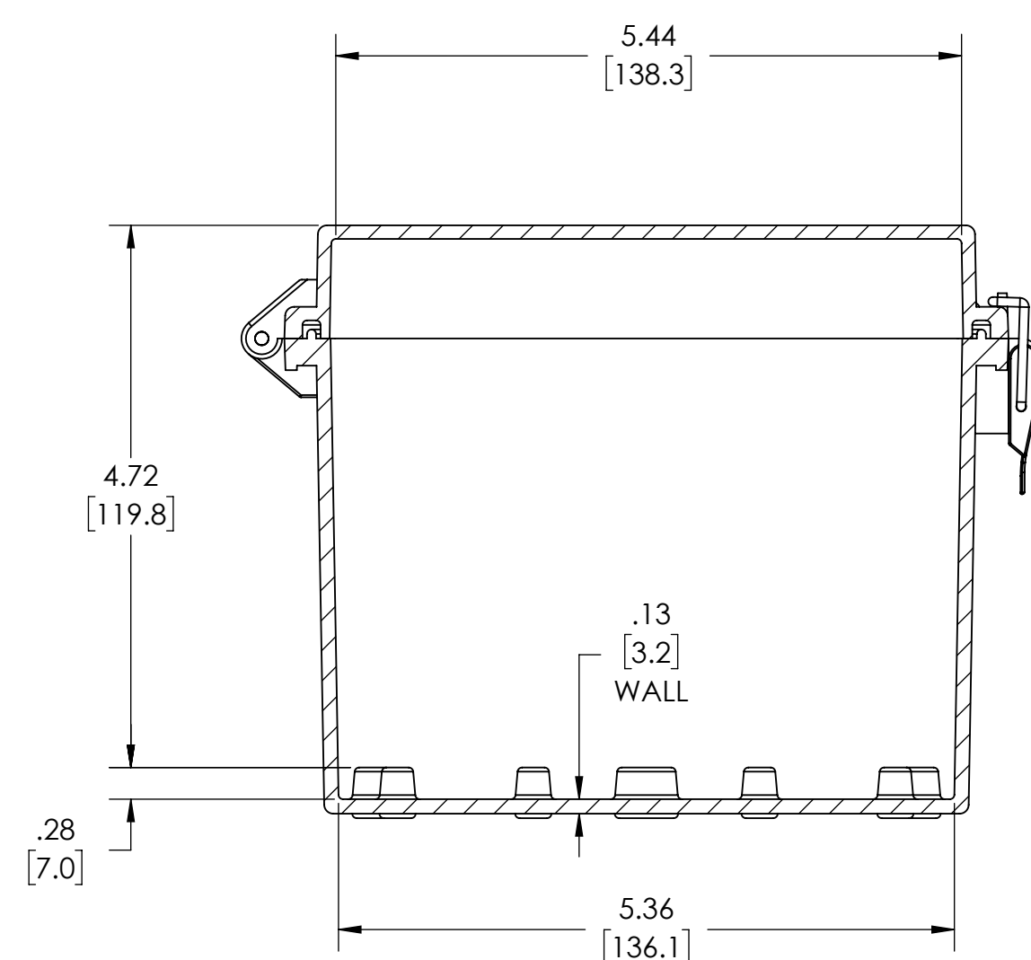
SECTION A-A
