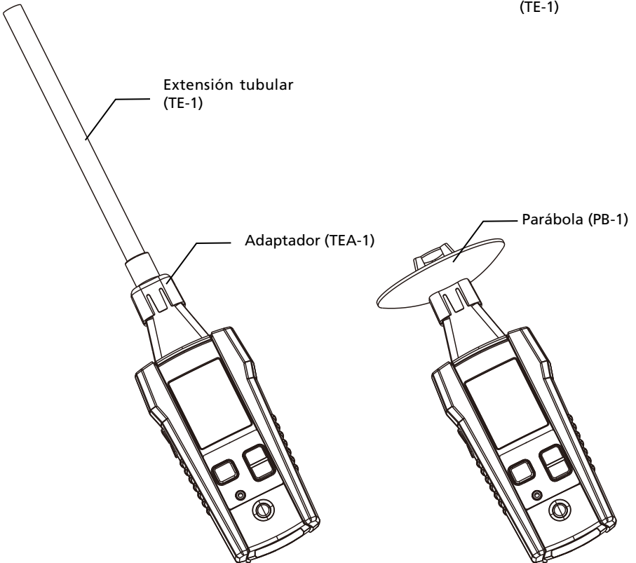
Figura 3.4: Accesorios ULD-400
