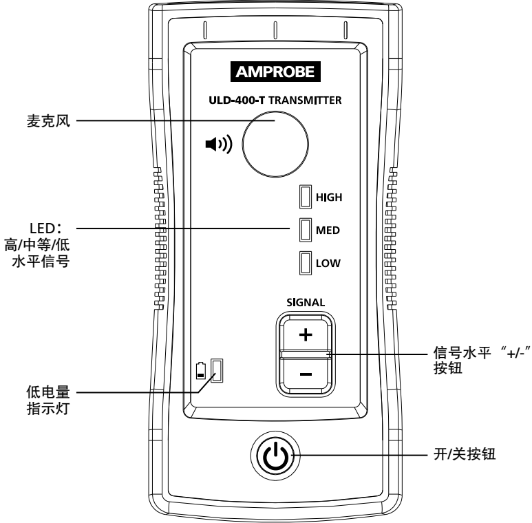
图3.3: ULD-400-T发送器
