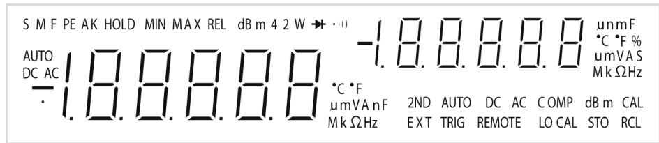
圖 1-1 照明所有區段的 VFD 全顯示器
