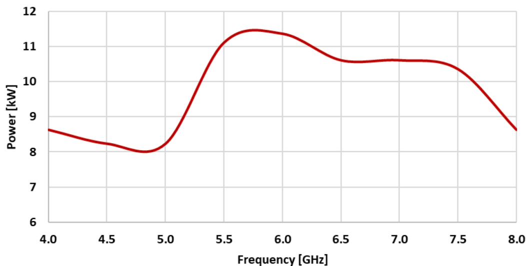
PTWT4G8G-8KW
