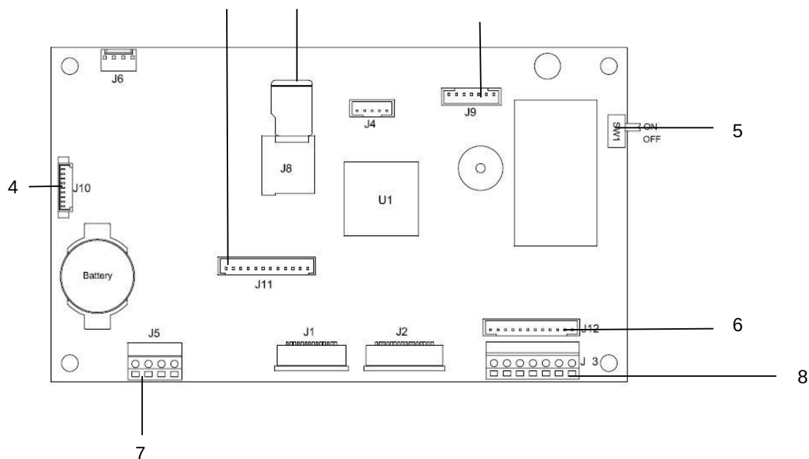
Abbildung 1-3 Hauptplatine
