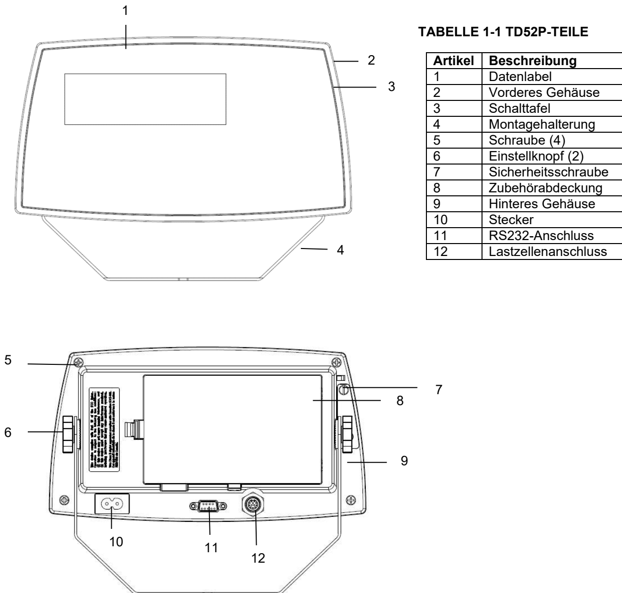
Abbildung 1-1 TD52P-Anzeige
