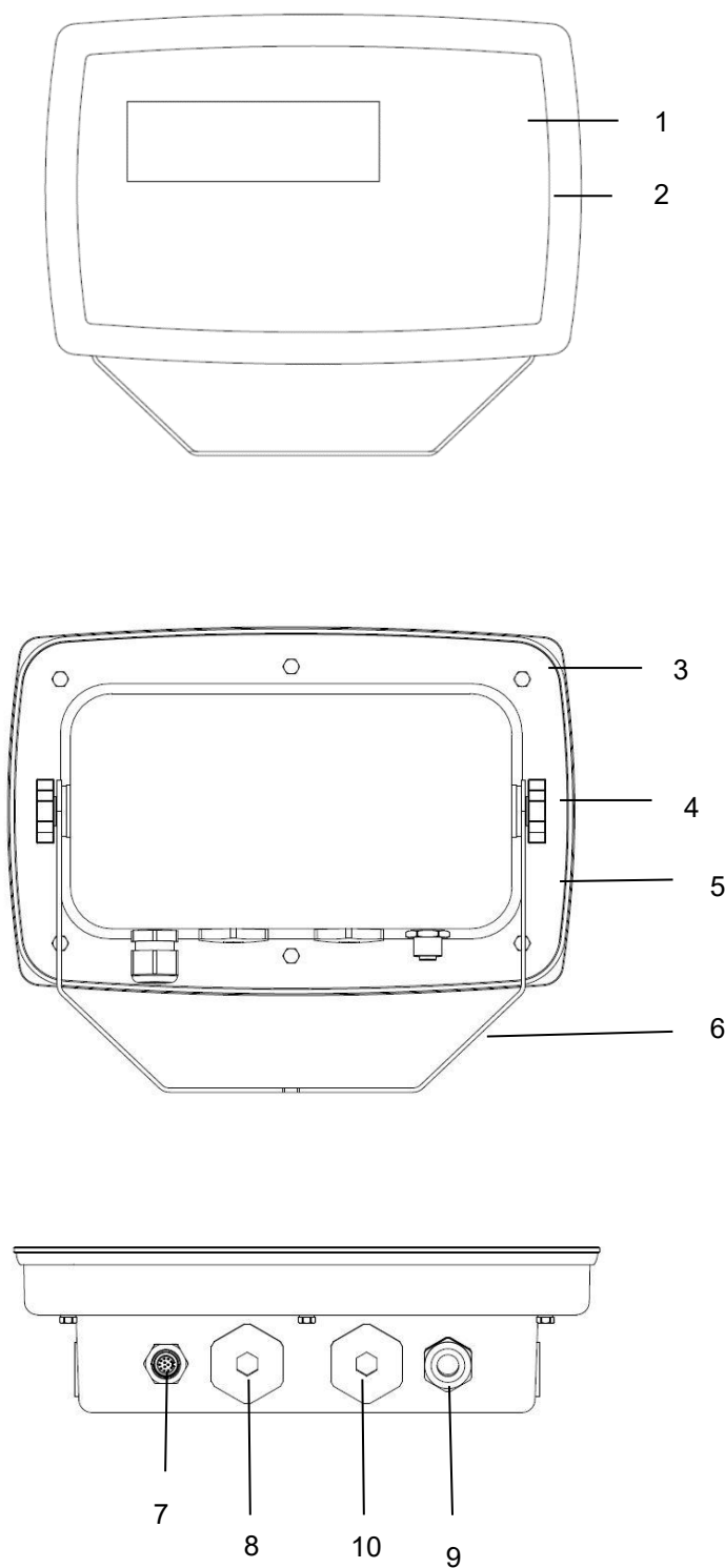
Figura 1-2 Indicatore TD52XW
