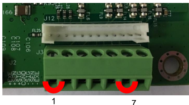
Figura 2-4 Collegamenti Ponticello
