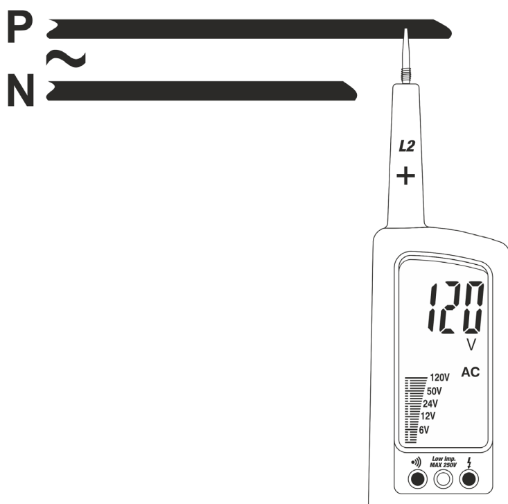
Fig. 5: Deteção de tensão AC 1-fio
