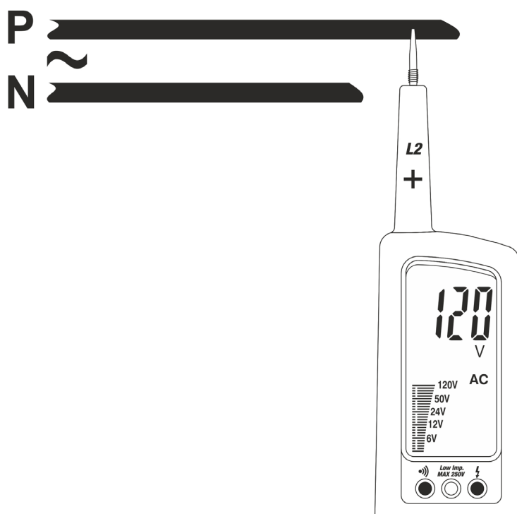
Fig. 5: Misura di Tensione AC a 1 filo (polarità)
