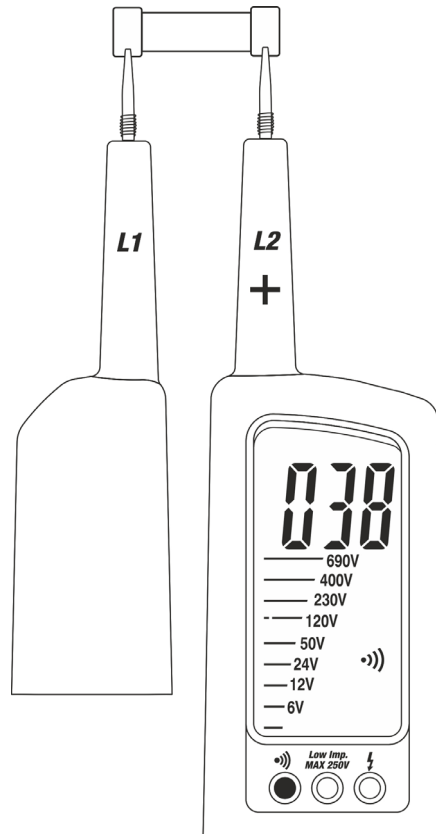
Abb. 7: Durchgangstest
