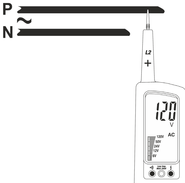
Abb. 5: Phasenprüfung einpolig
